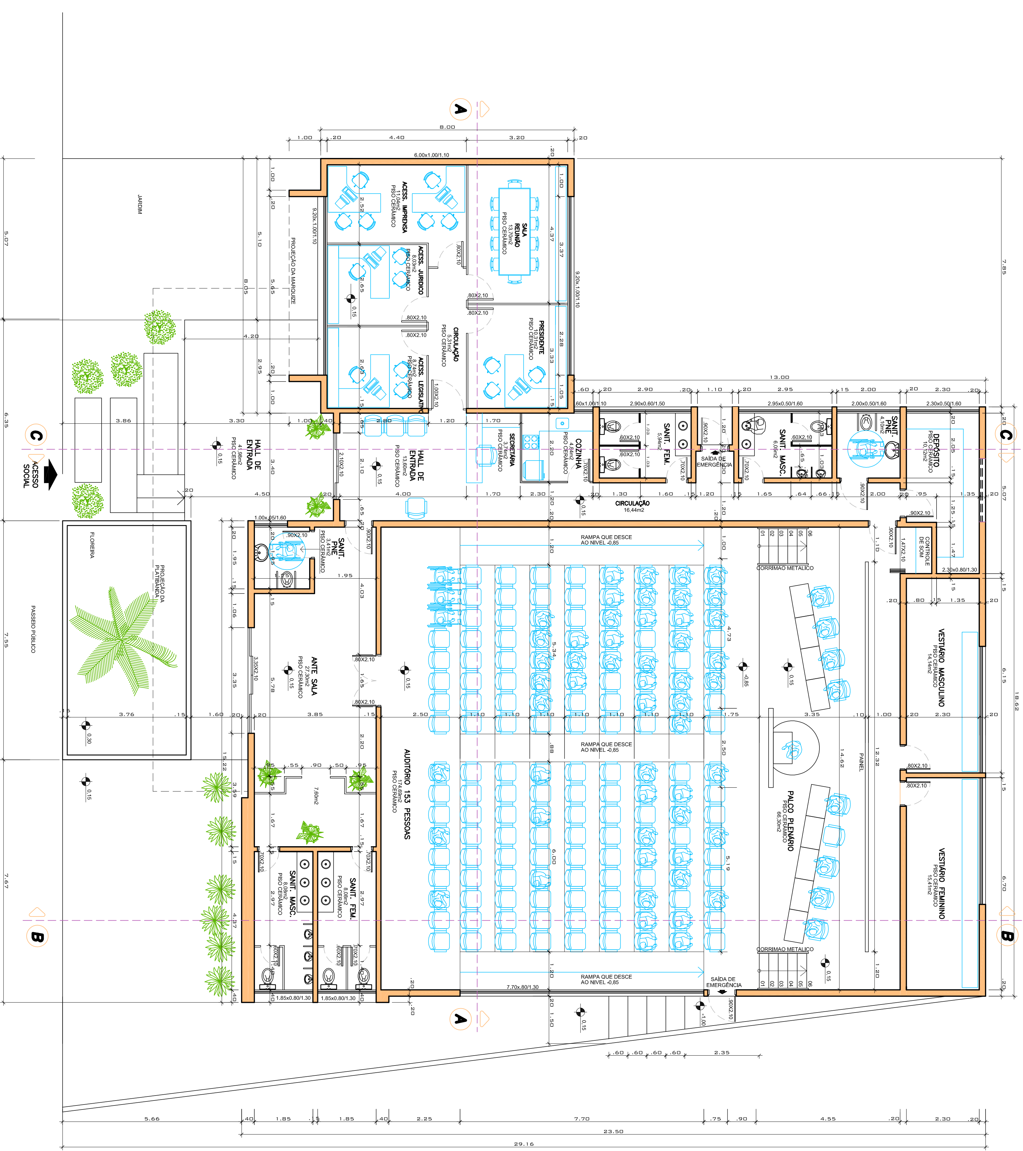
PLANTA BAIXA, escala : 1/75 ÁREA DO CONSTRUÍDA: 533,45 m2
